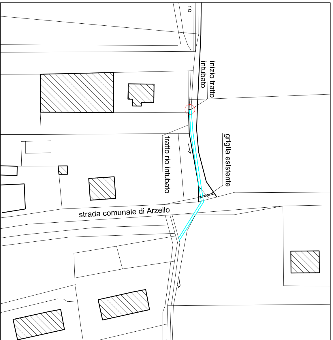
PLANIMETRIA - scala 1: 500
